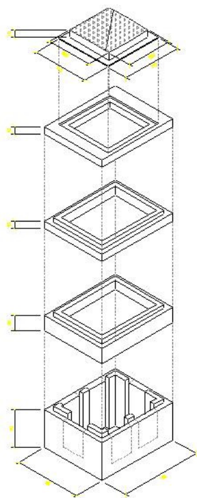
Figura 7 - Pozzetto 90x70: manufatti
