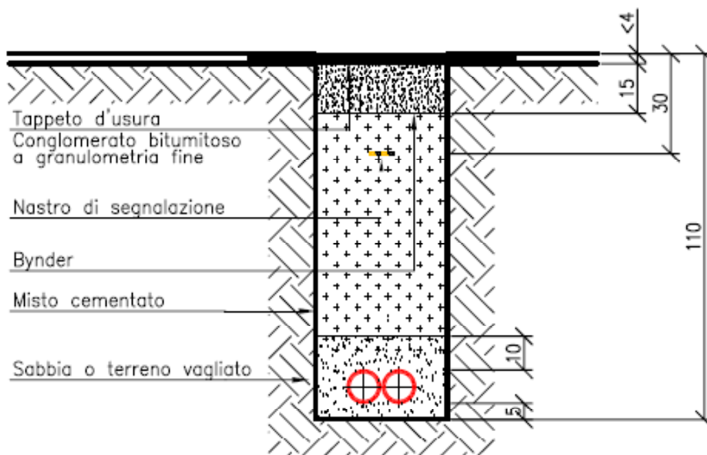
Figura 2 - Sezione tipo scavo tradizionale su strada
