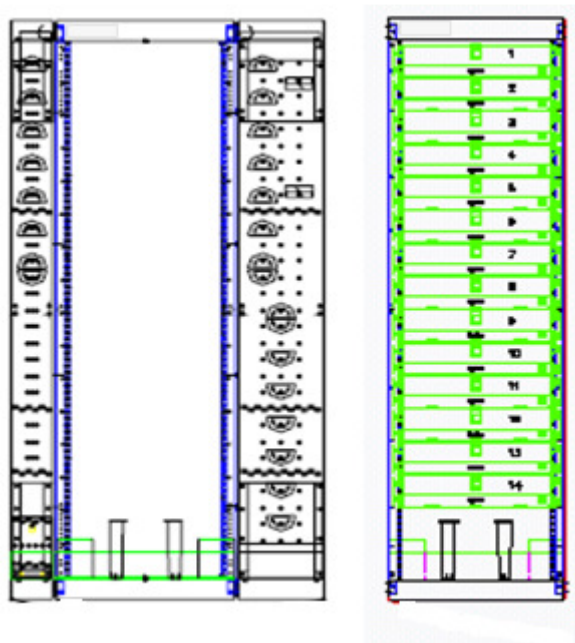
Figura 28 – Esempio telaio in tecnica N3
