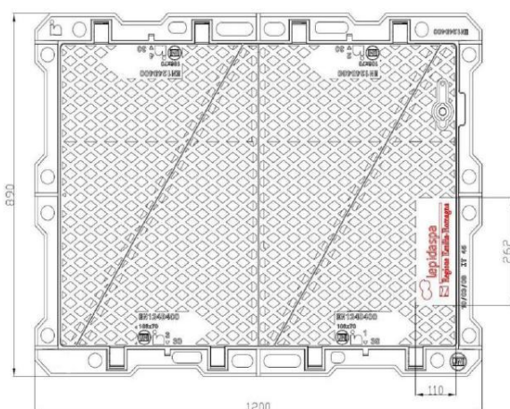
Figura 8 – Pozzetto 125x80: chiusini
