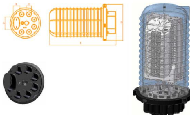
Figura 23 - Muffola
