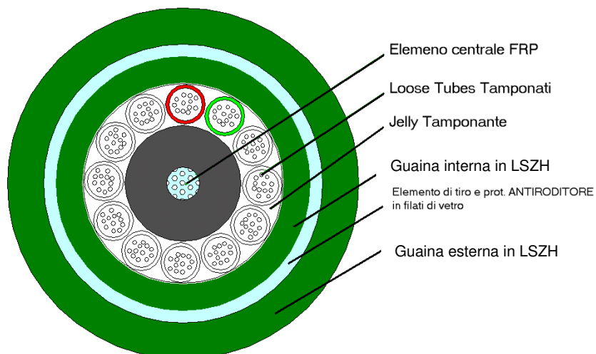
Figura 17 - Sezione di cavo a 144 fibre ottiche SMR con guaina LSZH
