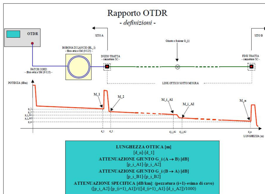
Figura 33 – Schema di misura: report OTDR
