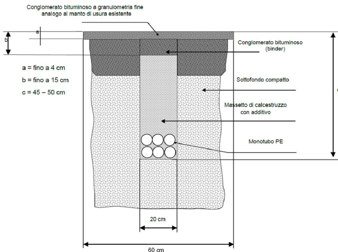
Figura 1 - Sezione tipo scavo in minitrincea
