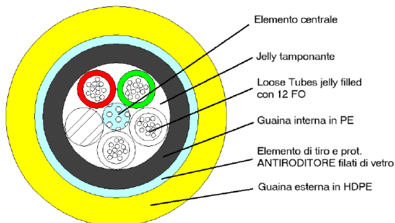
Figura 16 - Sezione di cavo a 48 fibre ottiche SMR (un tubetto riempitivo) e 24 fibre ottiche SMR (tre tubetti riempitivi) con guaina HDPE
