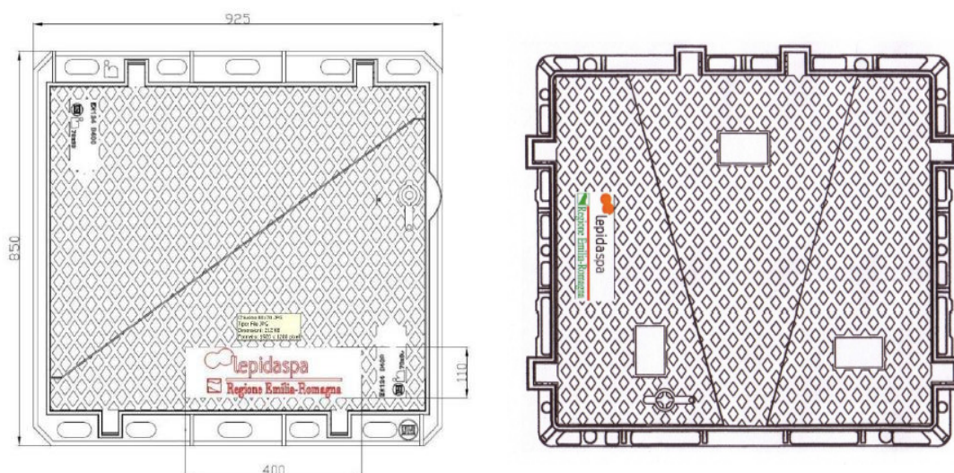
Figura 9 – Pozzetto 90x70: chiusini
