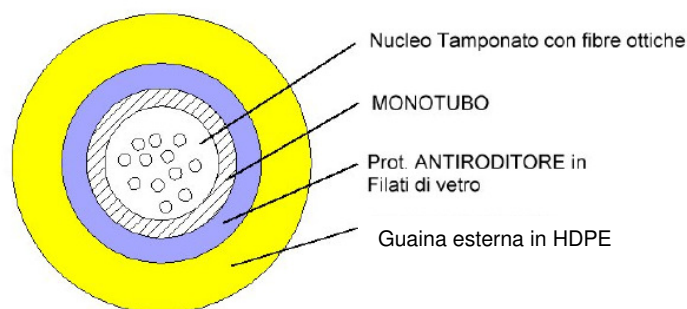
Figura 21 – Sezione di cavo a 12 fibre ottiche SMR con guaina in HDPE
