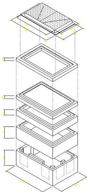
Figura 6 - Pozzetto 125x80: manufatti
