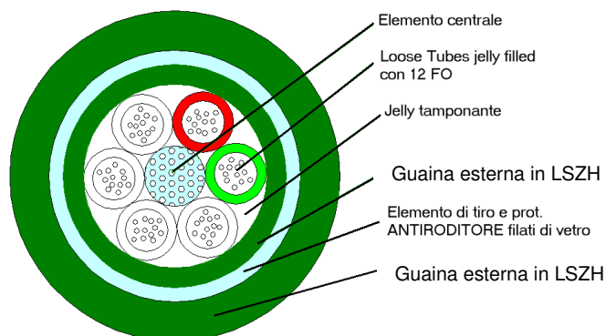
Figura 19 - Sezione di cavo a 72 fibre ottiche SMR con guaina LSZH
