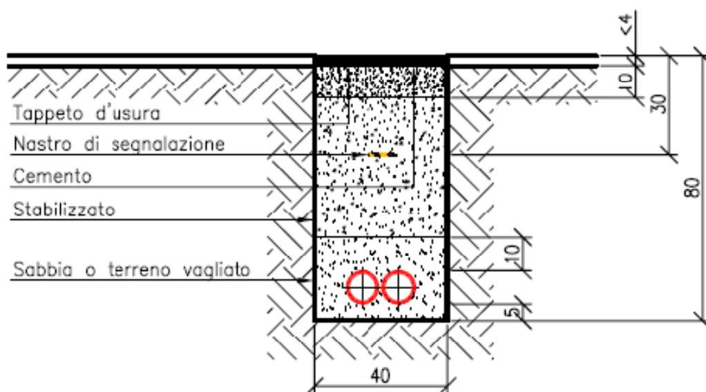
Figura 3 - Sezione tipo scavo tradizionale su marciapiede/pista ciclabile/area pedonale
