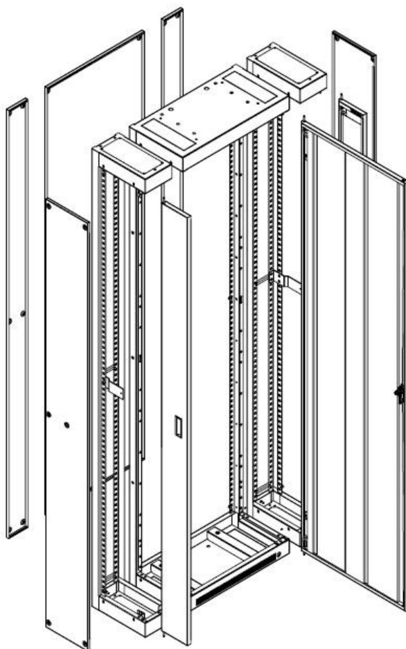
Figura 29 – Spaccato telaio N3
