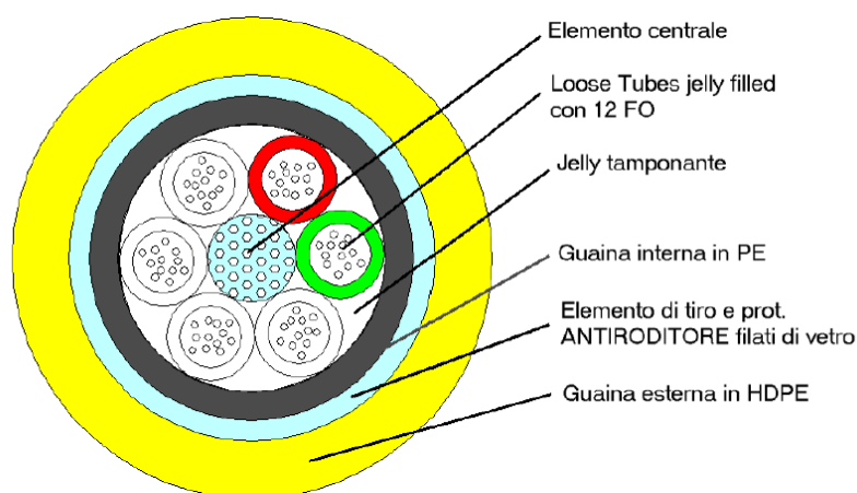
Figura 15 - Sezione di cavo a 72 fibre ottiche SMR con guaina HDPE
