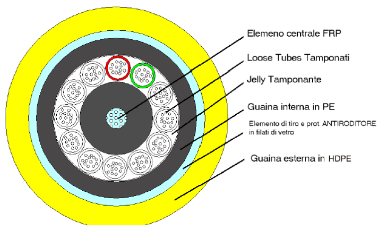
Figura 13 - Sezione di cavo a 144 fibre ottiche SMR con guaina HDPE
