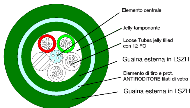
Figura 20 - Sezione di cavo a 48 fibre ottiche SMR (un tubetto riempitivo) e 24 fibre ottiche SMR (tre tubetti riempitivi) con guaina LSZH
