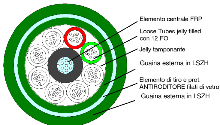
Figura 18 - Sezione di cavo a 96 fibre ottiche SMR con guaina LSZH
