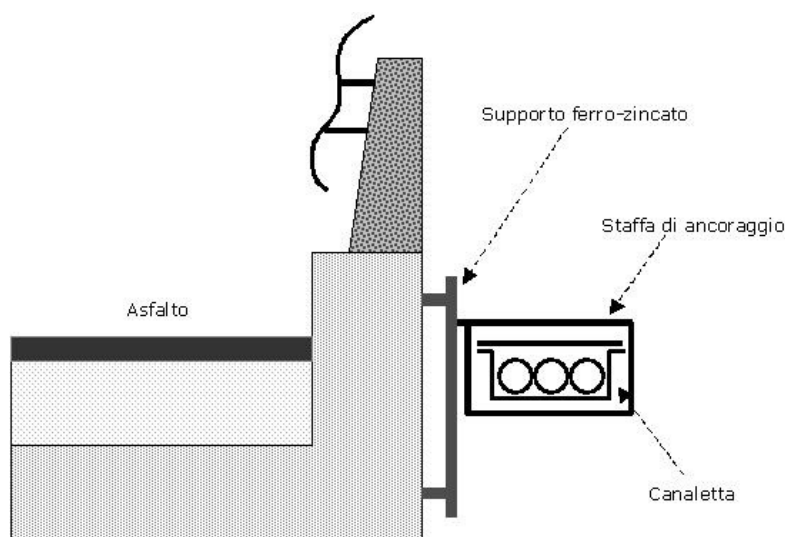
Figura 12 – Infrastrutture per attraversamento di ponti/viadotti
