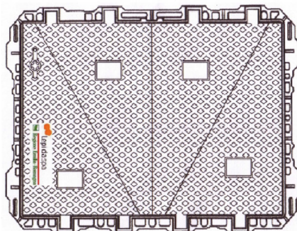
Figura 8 – Pozzetto 125x80: chiusini
