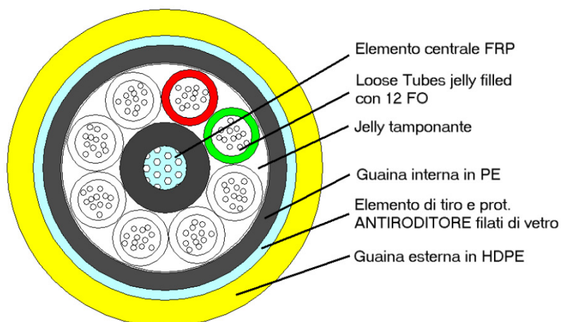
Figura 14 - Sezione di cavo a 96 fibre ottiche SMR con guaina HDPE
