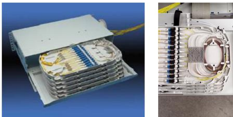
Figura 30 – Esempio di sub-telaio di giunzione/terminazione e particolare vassoio con interconnessioni LC/PC
