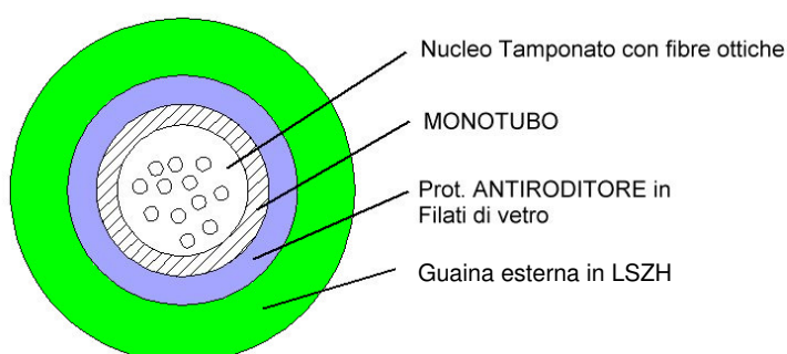
Figura 22 - Sezione di cavo a 12 fibre ottiche SMR con guaina LSZH
