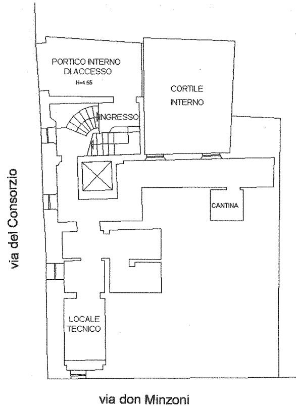
PIANO SEMITERRATO H= mt 2.40
