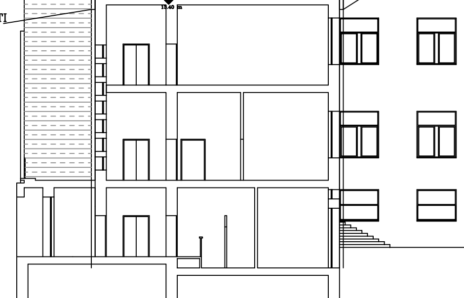
SEZIONE PROGETTO A-A SCALA 1:100
