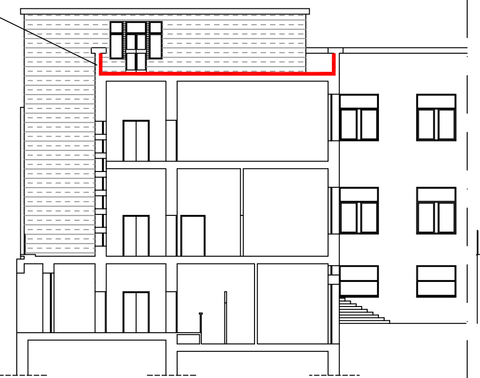
SEZIONE ESISTENTE A-A SCALA 1:100
