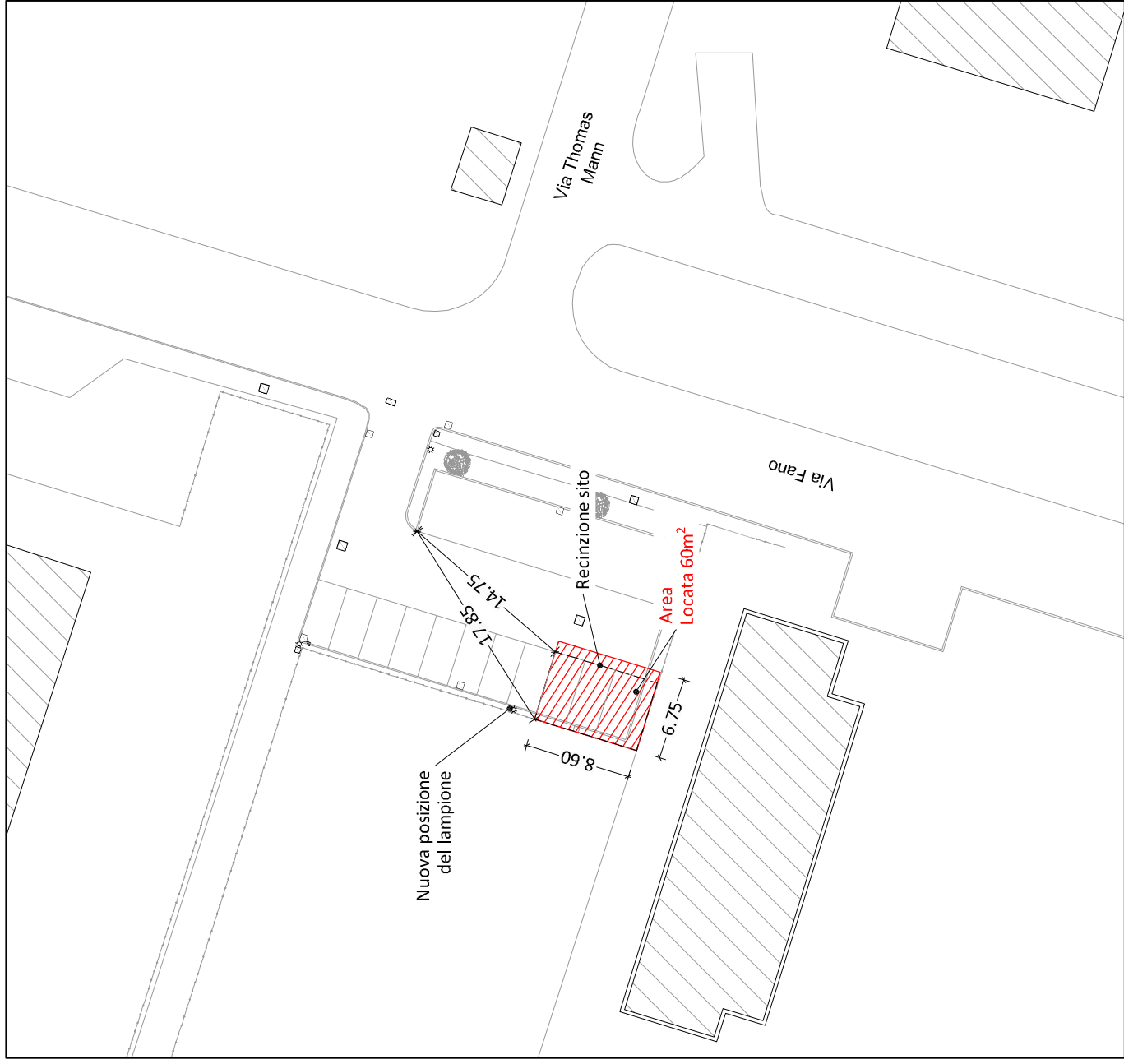
PLANIMETRIA - Scala 1:500
