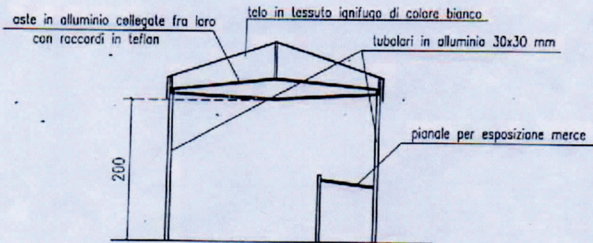
SEZIONE A:A 1:50
