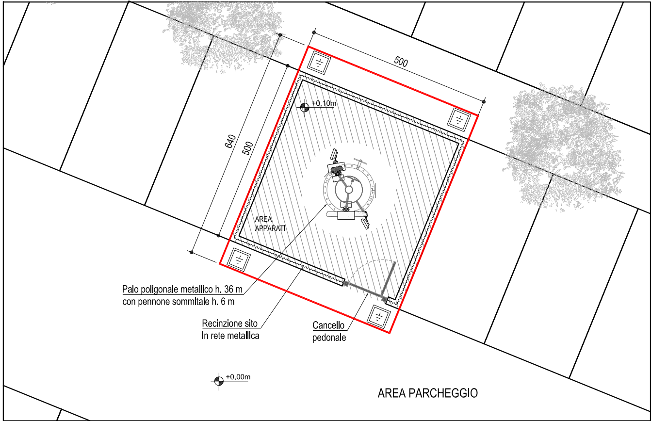
Pianta sito scala 1:100 - estratta dal Progetto di massima autorizzato
