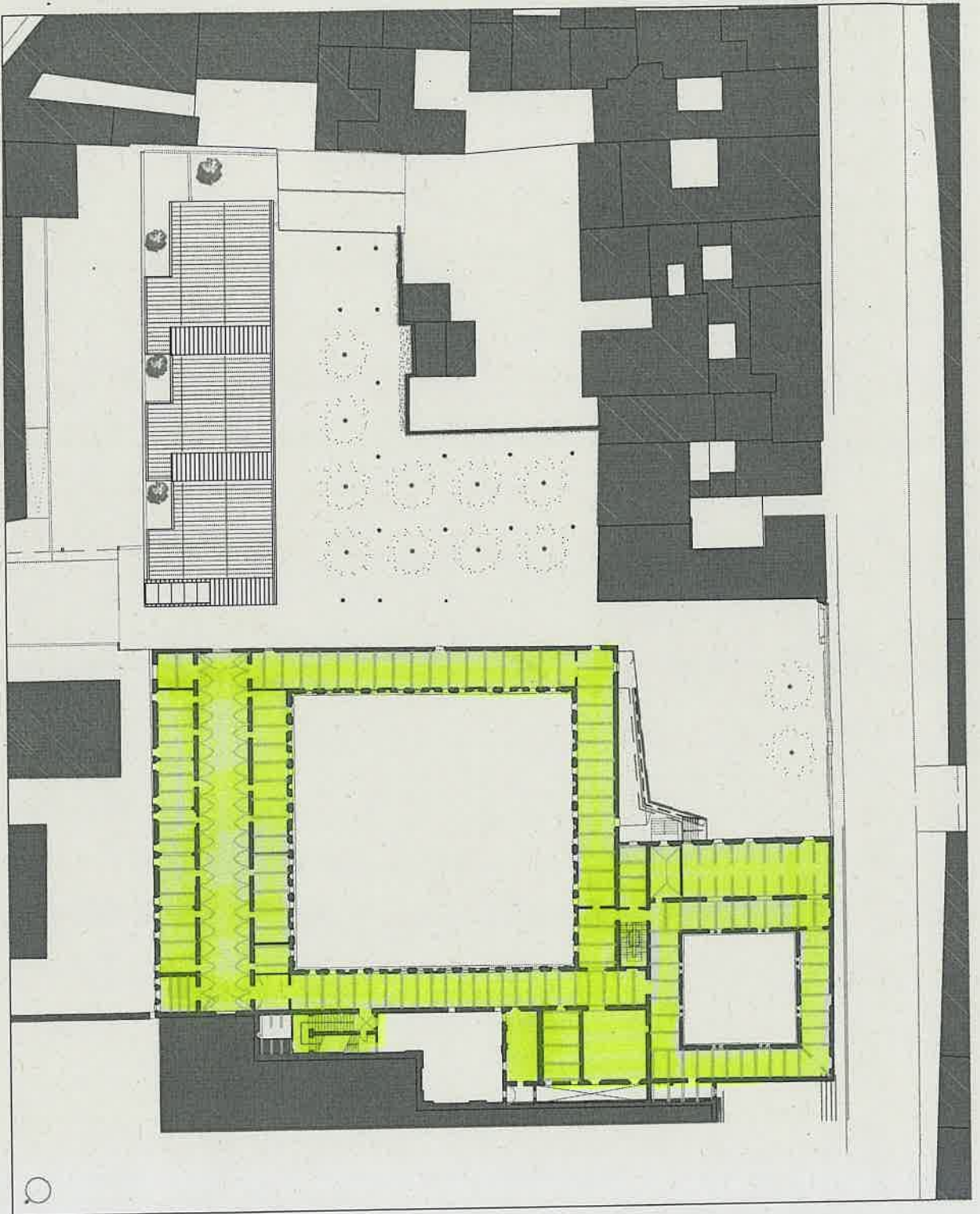
CHIOSTRI DI S.PIETRO PIANTA PIANO PRIMO
