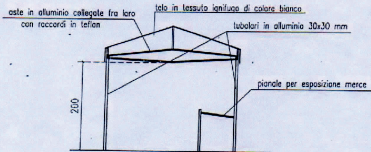
SEZIONE A:A 1:50
