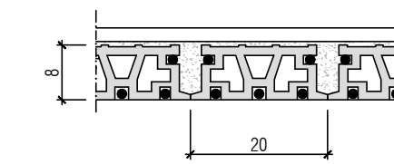
PARTICOLARE SOLAIO ESISTENTE SAP 8 Scala 1:10
