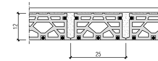
PARTICOLARE SOLAIO ESISTENTE SAP 12 Scala 1:10
