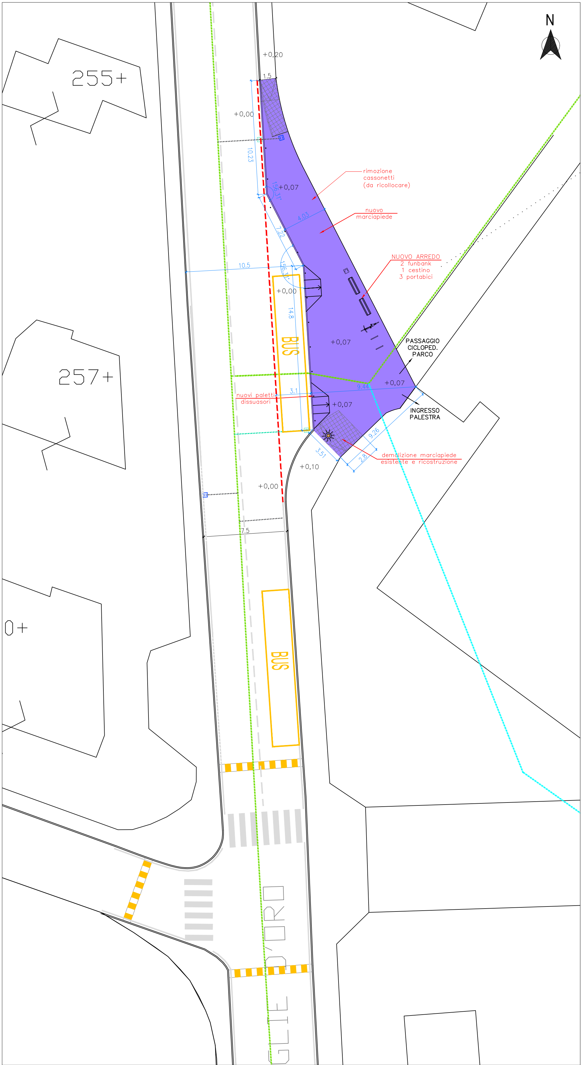
VIA MEDAGLIE D'ORO DELLA RESISTENZA STATO DI PROGETTO scala 1:200
