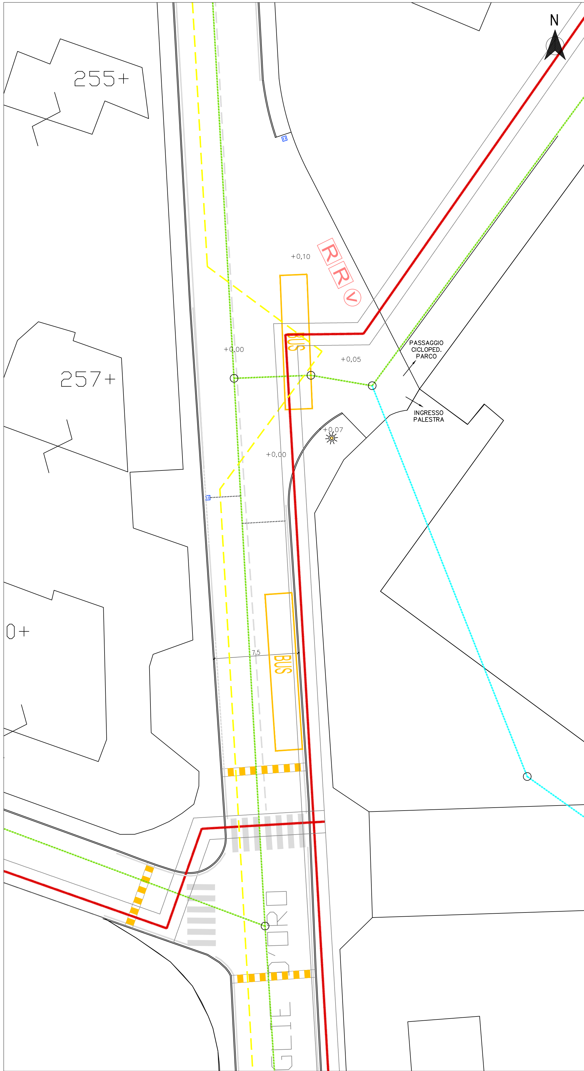
VIA MEDAGLIE D'ORO DELLA RESISTENZA STATO DI FATTO scala 1:200
