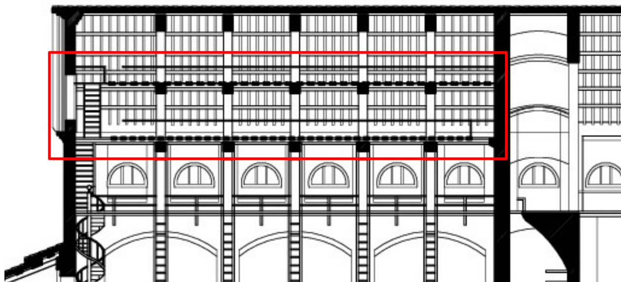
Attuale Localizzazione dei motori sulla graticcia
