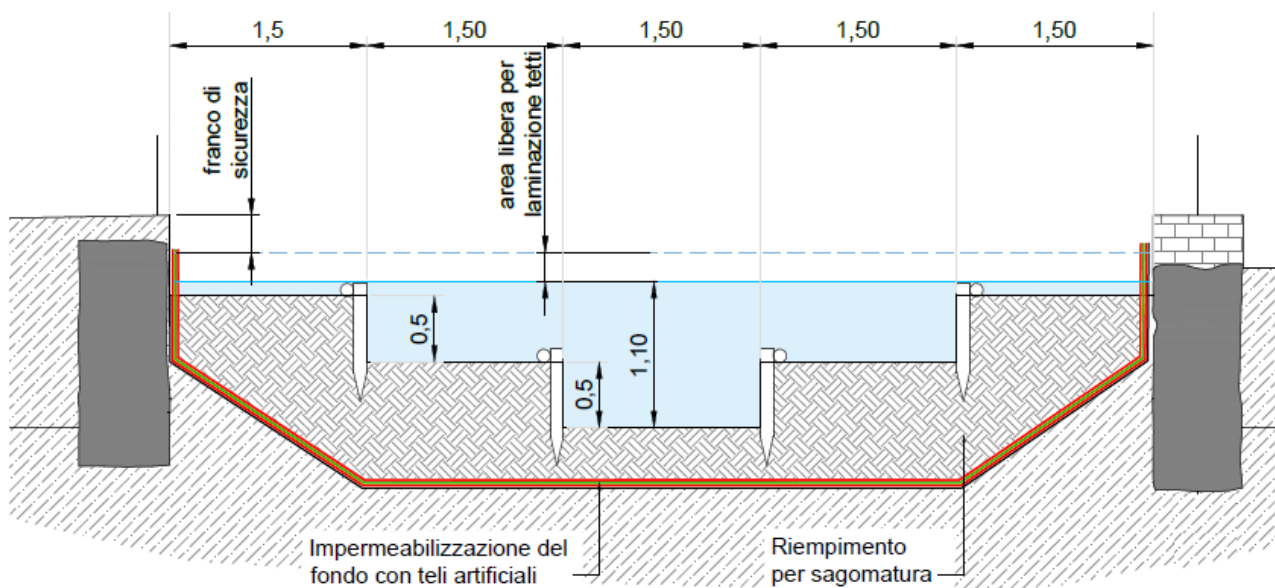
Fig. 16. Tipologica sezione canale in progetto
