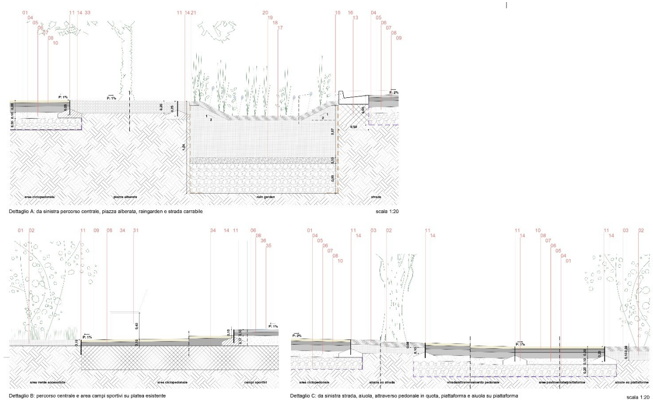
Figura 20 – Dettagli pavimentazioni.
