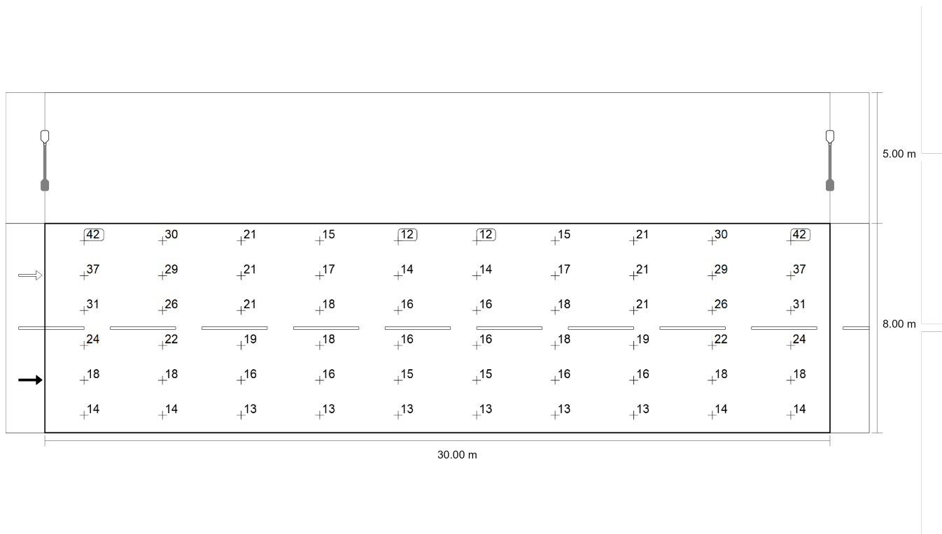
Valore di manutenzione illuminamento orizzontale [lx] (Raster dei valori)
