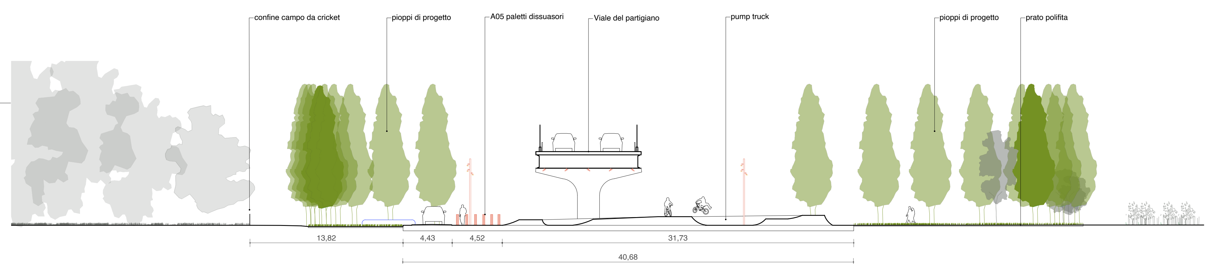
SEZIONE AA' PROGETTO scala 1:200
