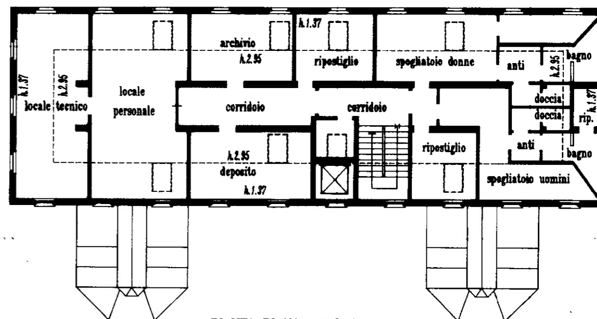
PIANTA PIANO SOTTOTETTO H m = 2.16 mt.
