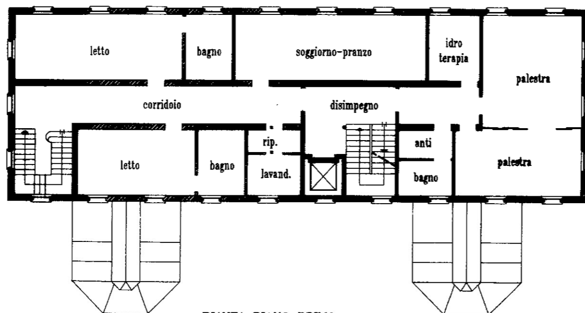
PIANTA PIANO PRIMO H = 3.20 mt.
