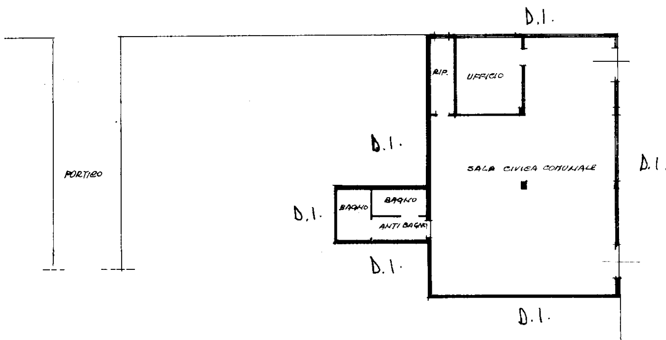
PIANTA PIANO TERRA H=300
